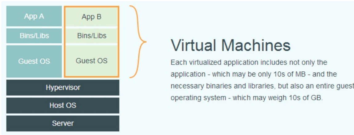
图 1.4.1.1 - 传统虚拟化
